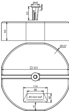
Maßbild BES 17KG M16 D337
