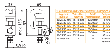
Maßbild UK 25 SK
