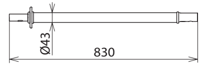
Maßbild H STK 43 800
