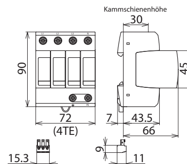
Maßbild DG M H TT 275 FM
