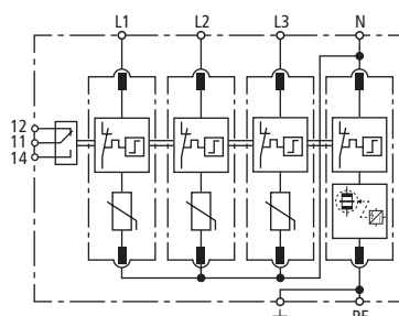
Prinzipschaltbild DG M H TT 275 FM
