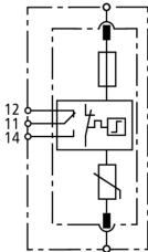
Prinzipschaltbild DG MOD E CI 440
