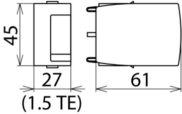
Maßbild DG MOD E CI 440
