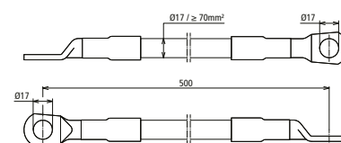
Maßbild D BEB 29 R / EBS 15-03-17
