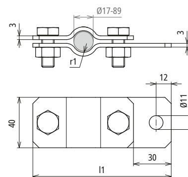
Maßbild ERS 34 AB11 STTZN
