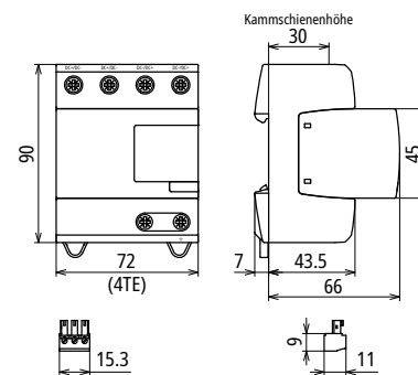
Maßbild DSE NG 2P 60 FM
