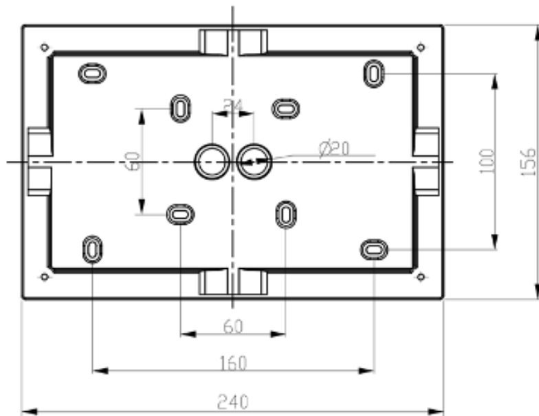
Maßzeichnung | dimensional drawing
