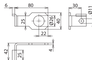
Maßbild AB EXFS IF1 W 26
