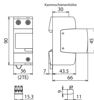
Maßbild DV M2 TT 2P 255 FM
