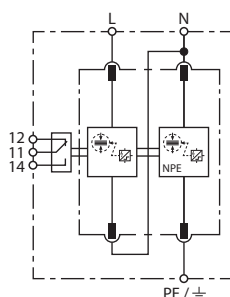
Prinzipschaltbild DV M2 TT 2P 255 FM
