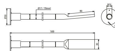
Maßbild D BEB 4 / EBS 15-03-19
