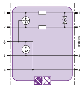
Prinzipschaltbild BXT ML2 BD DL S 15
