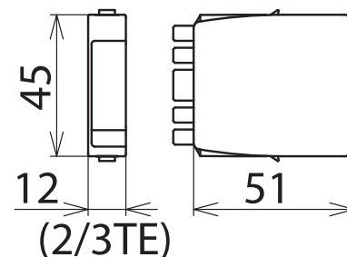
Maßbild BXT ML2 BD DL S 15
