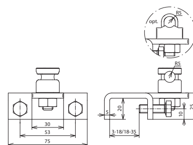
Maßbild AK 7.10 KSV W KBF18 35 STTZN
