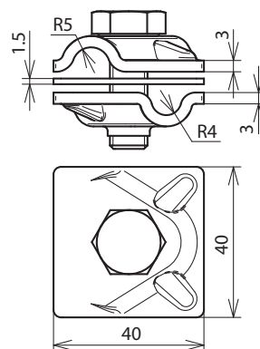
Maßbild ZMMVK 8 8.10 SKM10X30 CU AL
