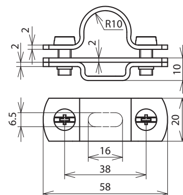
Maßbild LH ZS 20 H10 B6.5X16 V2A
