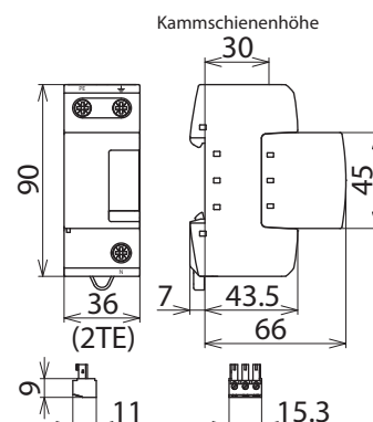
Maßbild DGPH M 255
