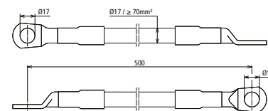
Maßbild D BEB 29 L / EBS 15-03-17
