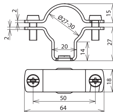
Maßbild LH ZS 27 GM8 V2A
