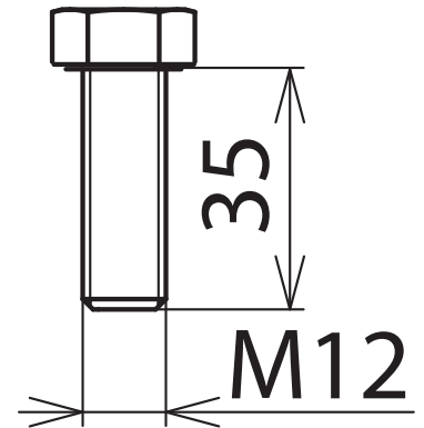
Maßbild SKS M12X35 V2A
