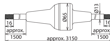
Maßbild EXFS KU
