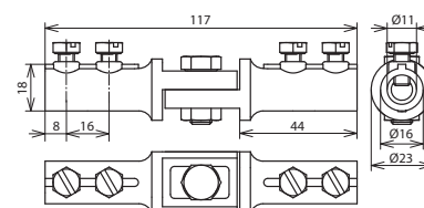
Maßbild OENTK 7.10 7.10 ZG
