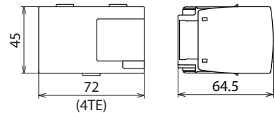
Maßbild DSE MOD NG 2P 60
