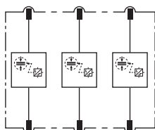
Prinzipschaltbild DSE MOD NG 2P 60
