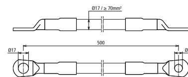
Maßbild D BEB 29-NF M12 M16 / EBS
