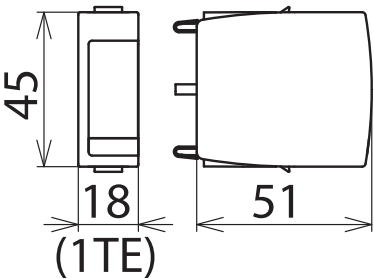
Maßbild DG MOD 275 VA
