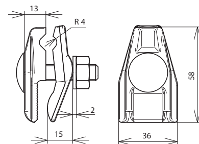
Maßbild AK 7.10 FRM10X45 KBF0.4 12 RG
