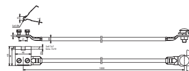
Maßbild ASSA D6 L1000 6.10 CU V2A
