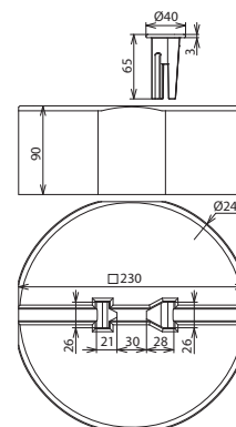
Maßbild BES 8.5KG M16 D240
