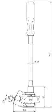
Maßbild EK I FL20 DGF
