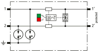
Prinzipschaltbild BCO MOD ML2 BD HF 24
