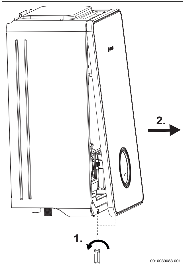
Bild 15 Frontplatten abnehmen
