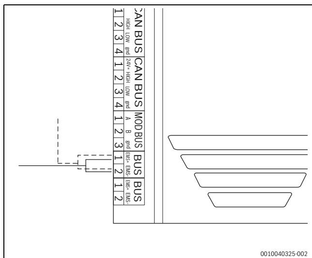
Bild 28 EMS-Anschluss
