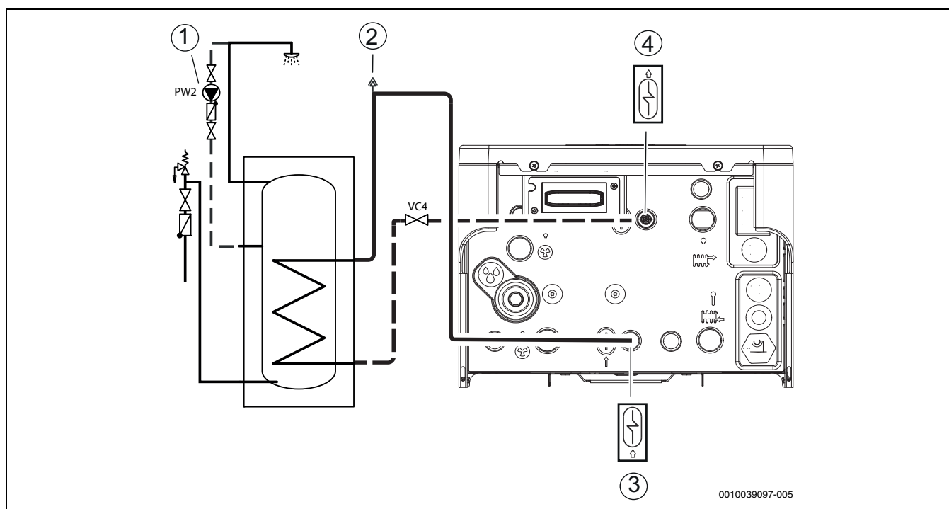
Bild 23 Trinkwasseranschlüsse Inneneinheit
