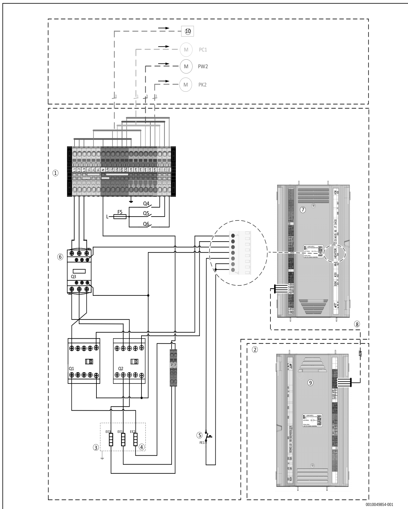
Bild 52 Spannungsversorgung Inneneinheit, Standard
