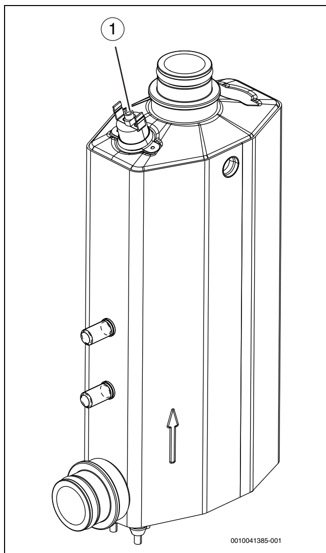
Bild 45 Elektrischer Zuheizer
