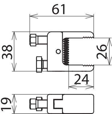
Maßbild KK M8 0 24 SK 10
