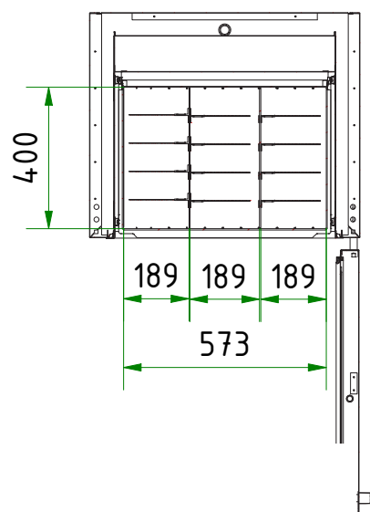
A-A ( 1 : 20 )
