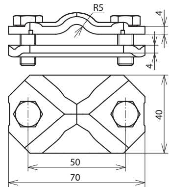
Maßbild VTK 7.10 FL30.40 STTZN
