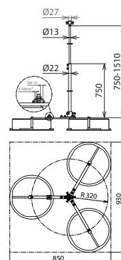
Maßbild V DBS RA320 PAE 27 V 750 1510 V2A
