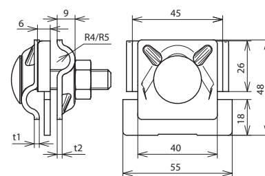
Maßbild FK MV 8.10 KBF0.7 10 CU
