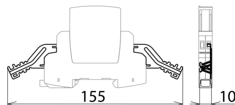
Maßbild SAK BXT LR
