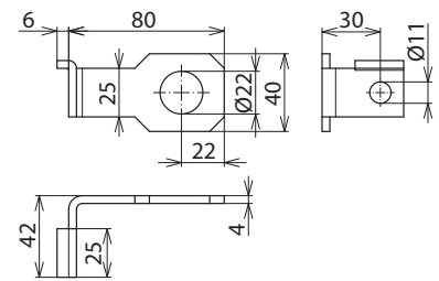
Maßbild AB EXFS IF1 W 22
