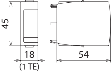
Maßbild DG MOD A NPE
