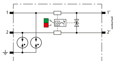
Prinzipschaltbild BCO MOD ML2 BD 180
