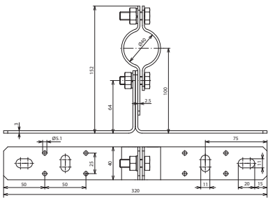
Maßbild WB D40 WA V2A
