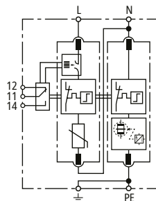
Prinzipschaltbild DG M TT 2P ACI 275 FM
