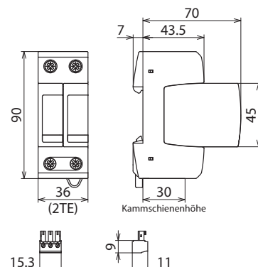
Maßbild DG M TT 2P ACI 275 FM
