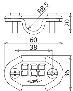
Maßbild NS 16 7SEG AL
