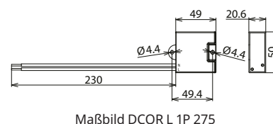
Maßbild DCOR L 1P 275
