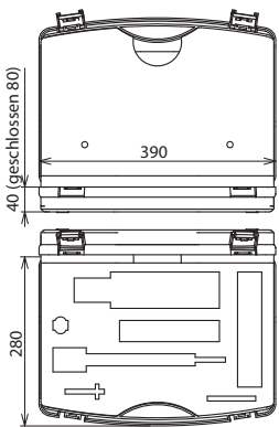
Maßbild KKL PK PHE3 L
