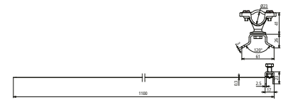
Maßbild LH ZS 23 SB50.300 PA V2A
