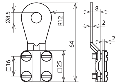
Maßbild EKSG 8 AQ6 16 CUGALZN
