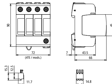
Maßbild DG MD TT 150 FM
