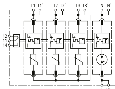
Prinzipschaltbild DG MD TT 150 FM
