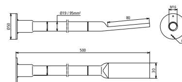
Maßbild D BEB 5-FLEX / EBS 15-03-19
