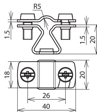
Maßbild LH ZS 8.10 FL20 M8 CU
